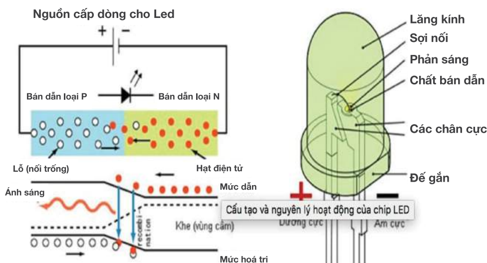
Cấu tạo và nguyên lý hoạt động của chip led
